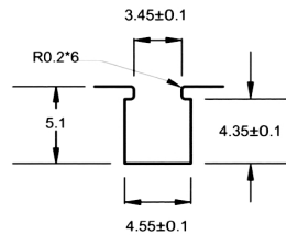
沟槽尺寸图
