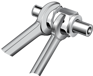
5. 用扳手握住公螺母，将母螺母拧1/8圈
