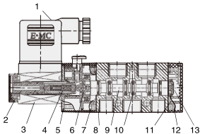
单电控电磁阀
