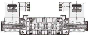
双电控电磁阀
