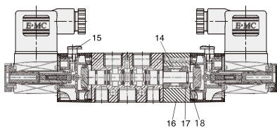
三位置电磁阀
